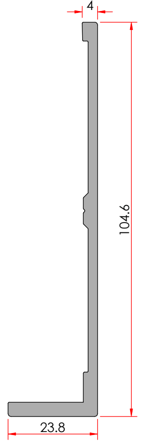
L-Üst Bağlantı Profili L-Top Connection Profile
